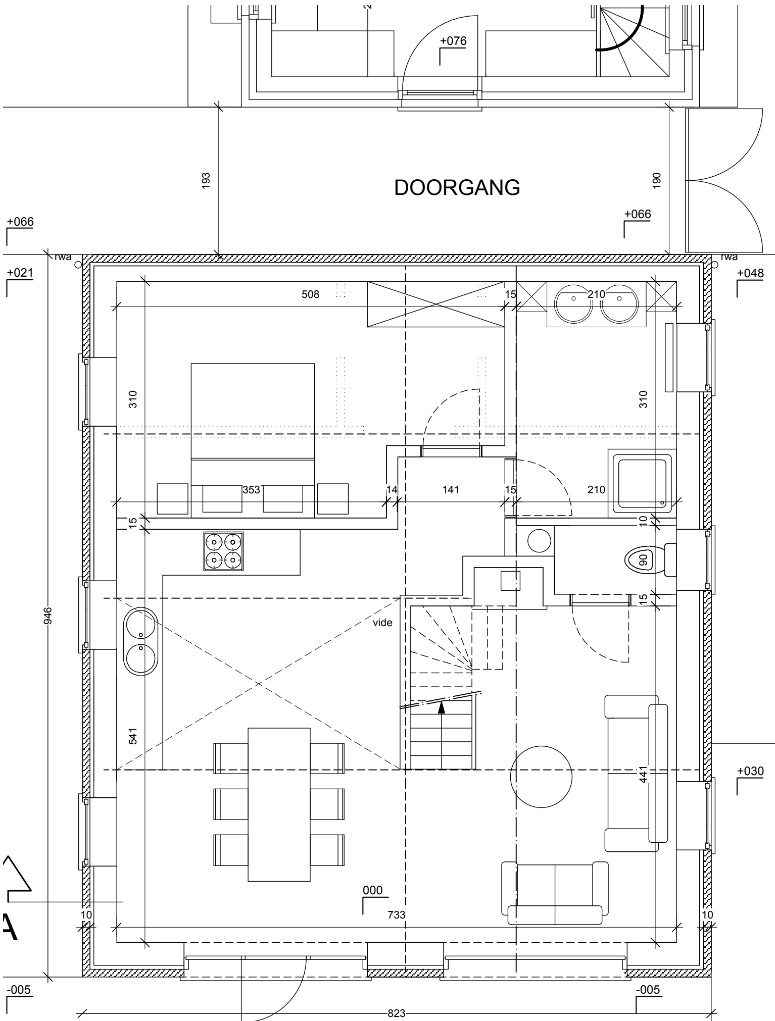
PLAN GELIJKVLOERS nieuw
